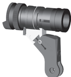
Figura 13: Portamirino universale per F ass 57 (montaggio normale), diversi modelli
