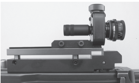
Bild 16: Dioptraträger zu Stgw 57 zur Aufnahme schussfester Diopter, diverse Fabrikate
