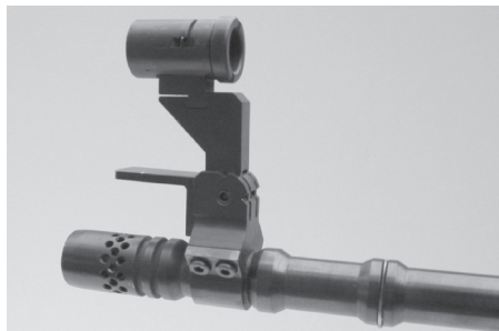
Figure 14: Bloc guidon comme rallongement de la ligne de visée (montage sur canon), produits divers
